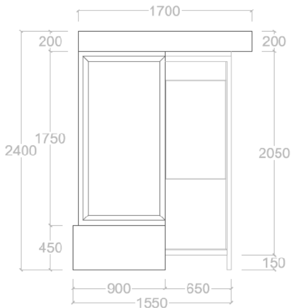
Bočni izgled (levo)
