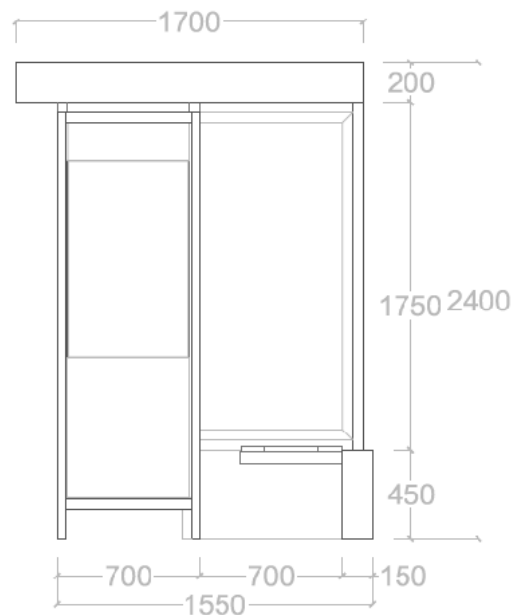
Bočni izgled (desno)
